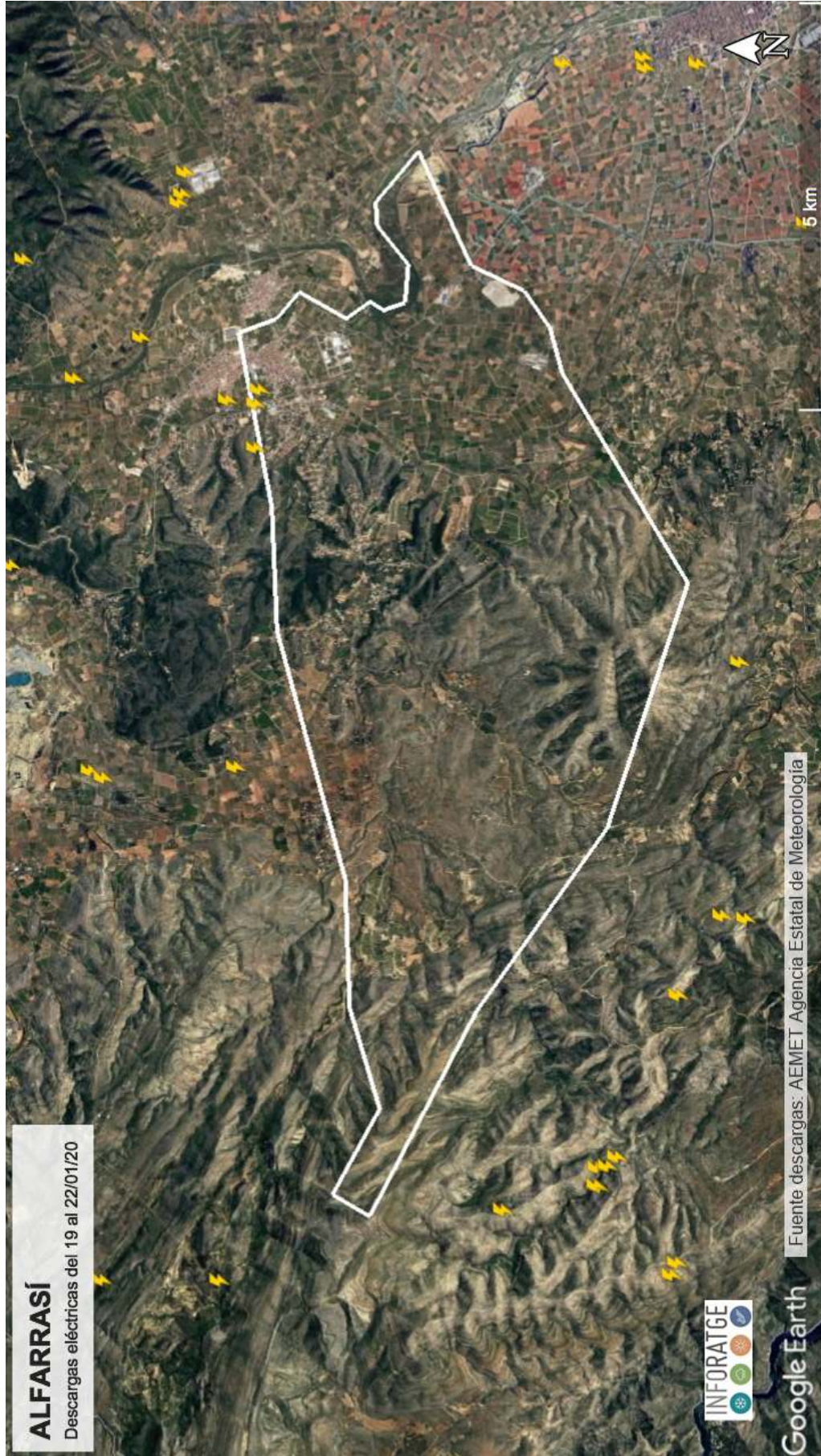
Geolocalización de las descargas eléctricas nube-tierra registradas en el término municipal de CATADAU y alrededores entre el 19 y el 22/01/20 Fuente descargas: AEMET Agencia Estatal de Meteorología
