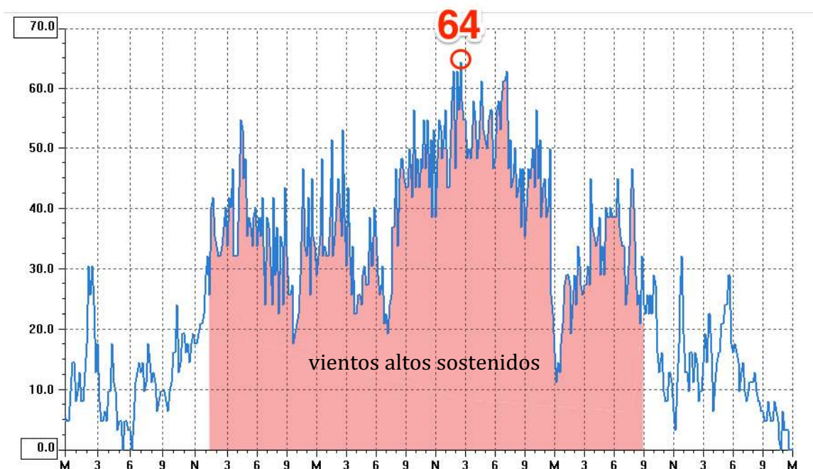
Ráfagas de viento registradas por la estación municipal de CATADAU (centro localidad) entre el 19 y el 21/01/20 (en km/h)
