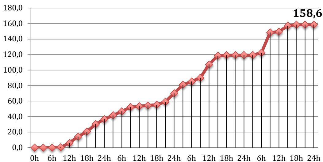
Evolución lluvia acumulada en CATADAU (Urb. Llama Molina) del día 19 al 22/01/20 en períodos de 3 horas (en l/m 2 )
